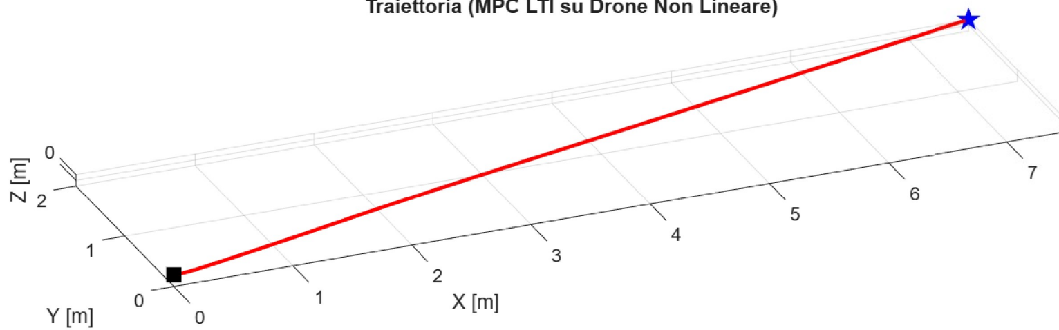
Traiettoria (MPC LTI su Drone Non Lineare)
